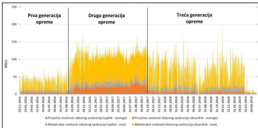
Slika 1. Vremenska serija dobijena procesom monitoringa tri generacije mrežne opreme
